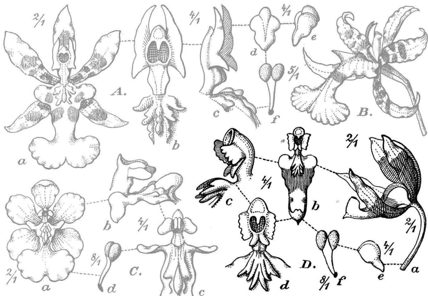
Fig. 24. A: a—f Oncidium drepanopterum Kränzl.*) a flos \frac{2}{1} , b et c gynostemium c. basi labelli, d et e anthera, f pollinium. — B: a O. trinasutum Kränzl. a flos. — C: a—d O. helicanthum Kränzl. a flos vi expansus. b gynostemium c. basi labelli a latere visum, c id. a fronte visum, d pollinium. — D: a—f O. lintricus Kränzl. a flos \frac{2}{1} , b gynostemium a fronte, c id. a latere visum, d id. cum crista labelli, e anthera, f pollinium.
